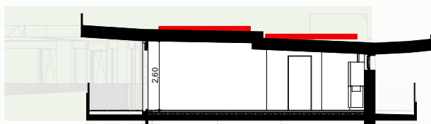
Schnitt Deckensprung
